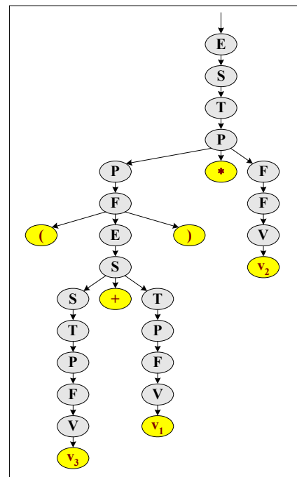
Σχήμα: Γραμματική για αλγεβρικές εκφράσεις, και συντακτικό δένδρο για την έκφραση: (v_3 + v_1) * v_2 .
