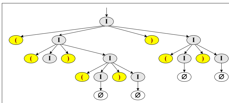
Σχήμα: (Το) συντακτικό δένδρο για την λέξη « ((()())()) » της γλώσσας L(G_{\text{ππ}}) .
