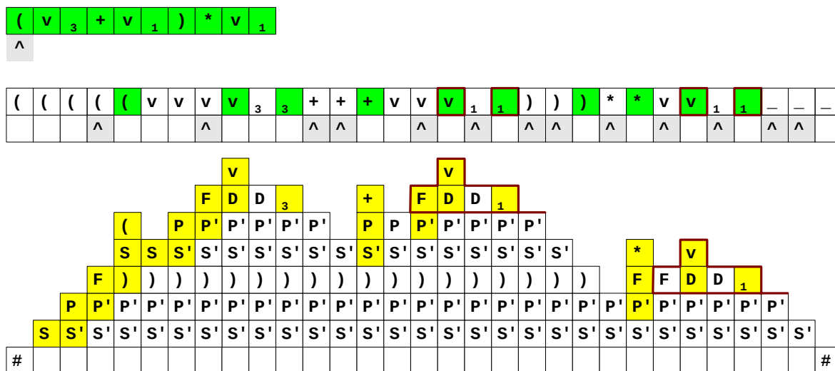
Σχήμα: Η εξέλιξη της στοίβας κατά την ανάλυση της έκφρασης (v_3 + v_1) * v_1 .
